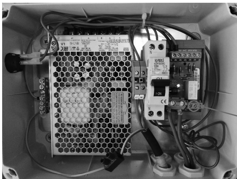
Modèle de coffret pour volet
